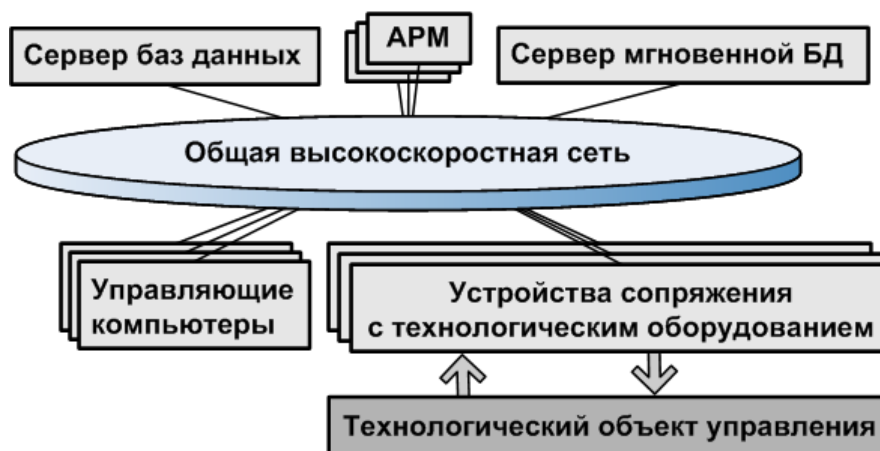
Рисунок 2 – Новая архитектура АСУТП
