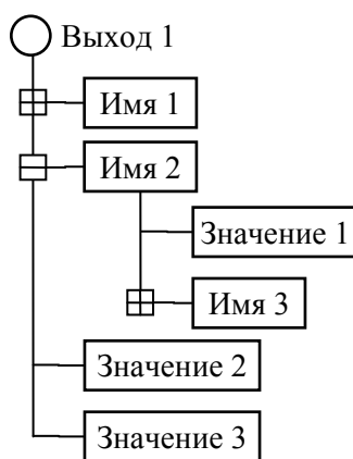
Рис. 2. Древоподобная структура данных
