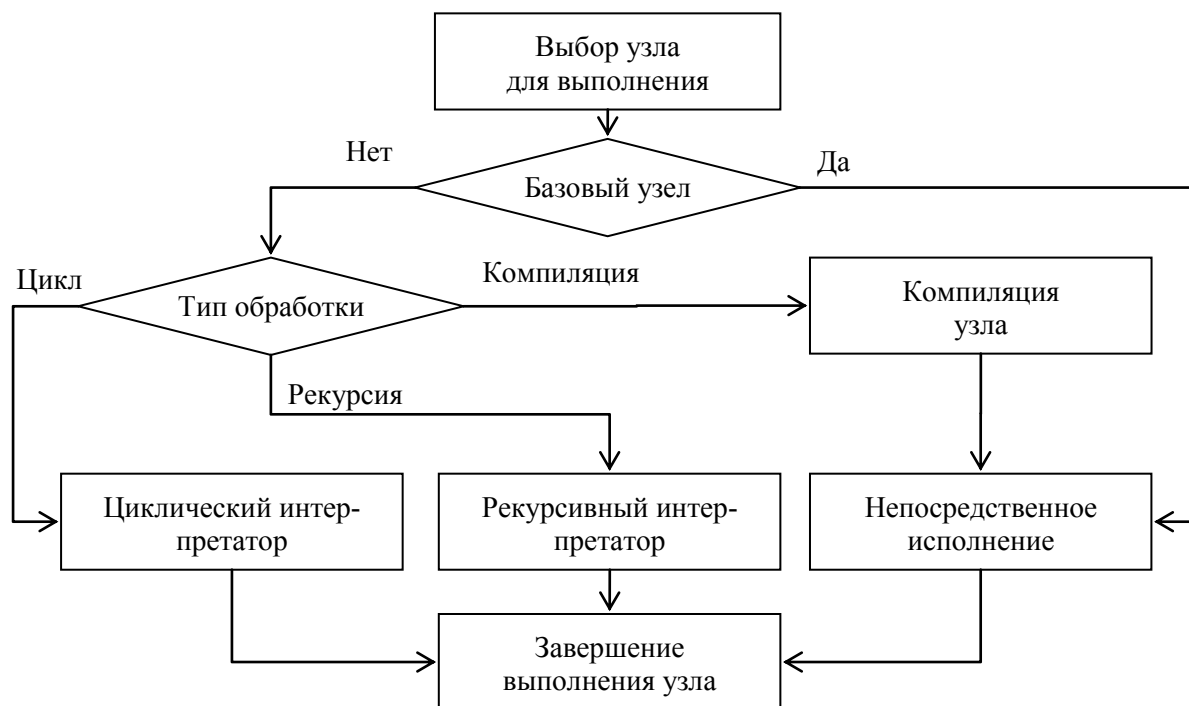
Рис. 3. Выполнение узла совмещённой модели
